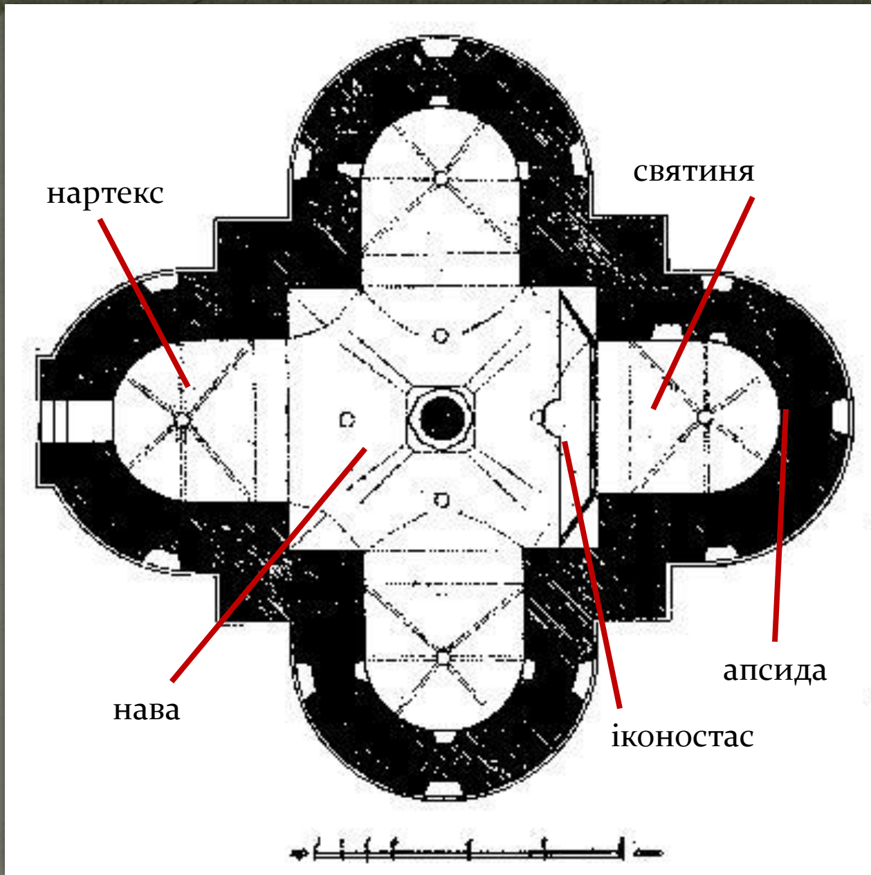
➤ Церква Покрову Пресвятої Богородиці, план, 1476.
