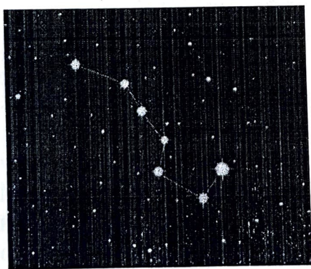
Сузір'я Зоряний Віз
